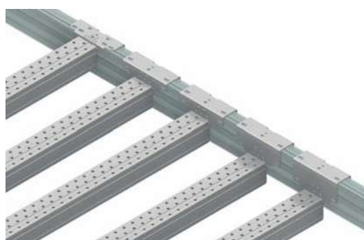
14 Rompitratte 70 x 70 modulari - filo corrente o ribassati
