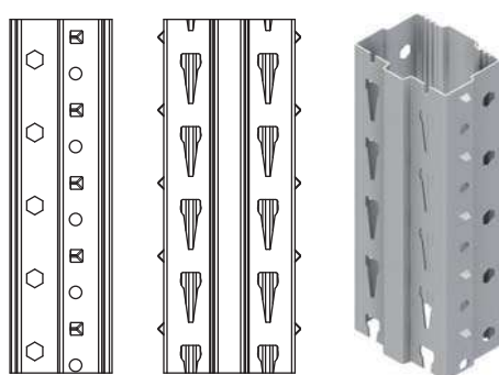
1 Montante Superbo
