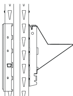
20 Guida DRIVE-IN su staffa singola e doppia
