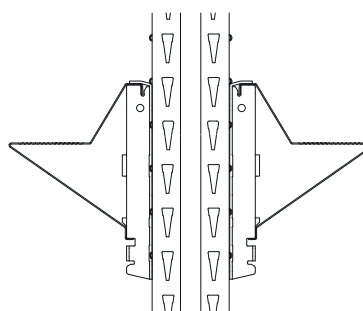
21 Guida DRIVE-IN bifronte su staffa singola
