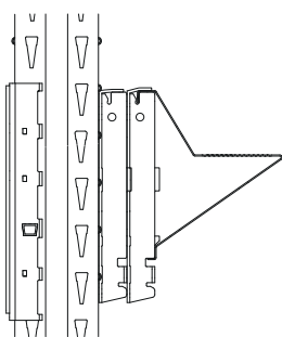
20 Guida DRIVE-IN su staffa singola e doppia
